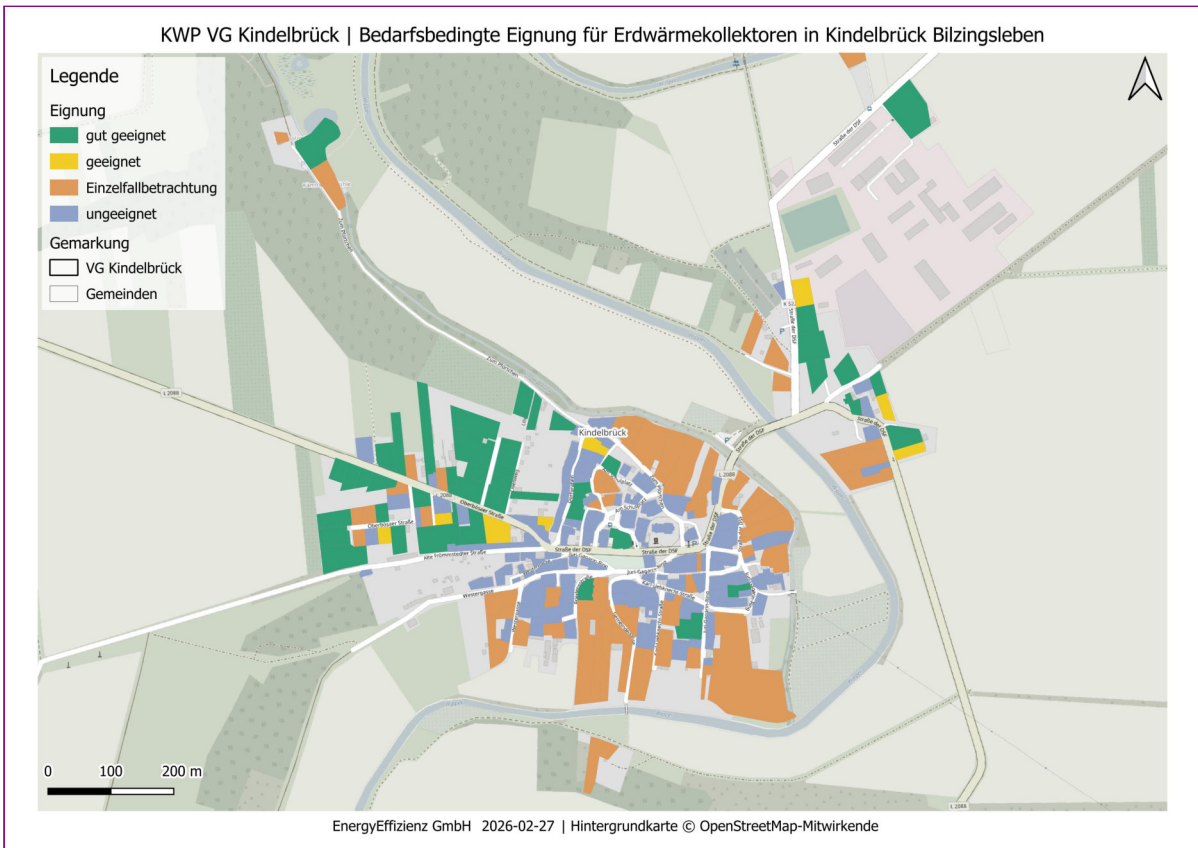
Abbildung Anhang 38: Landgemeinde Kindelbrück: Ortsteil Bilzingsleben: Bedarfsbedingte Eignung von Erdwärmekollektoren auf Flurstücksebene
