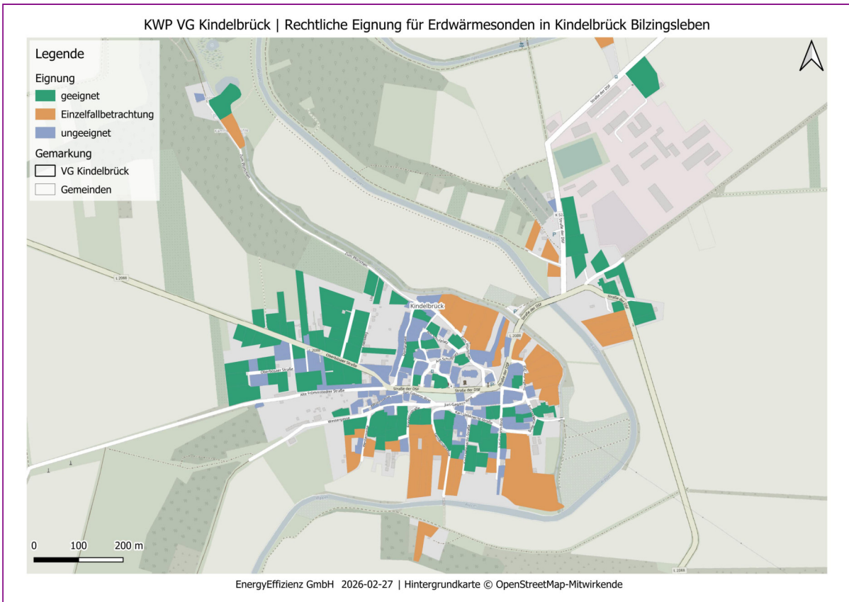
Abbildung Anhang 39: Landgemeinde Kindelbrück: Ortsteil Bilzingsleben: Rechtliche Eignung von Erdwärmesonden auf Flurstücksebene
