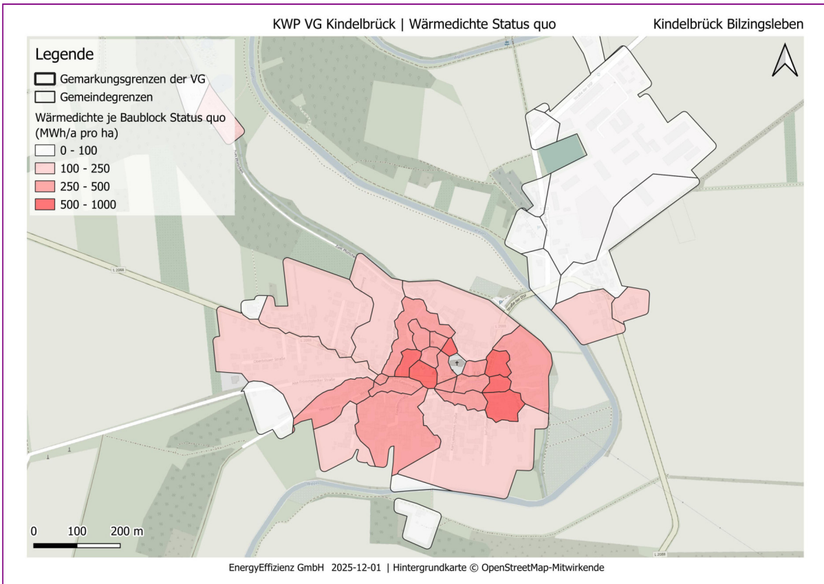
Abbildung Anhang 34: Landgemeinde Kindelbrück: Ortsteil Bilzingsleben: Wärmedichte je Baublock im Status quo
