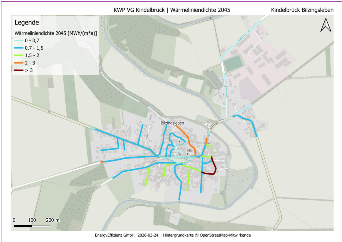
Abbildung Anhang 36: Landgemeinde Kindelbrück: Ortsteil Bilzingsleben: Wärmelinienichte im Zieljahr 2045
