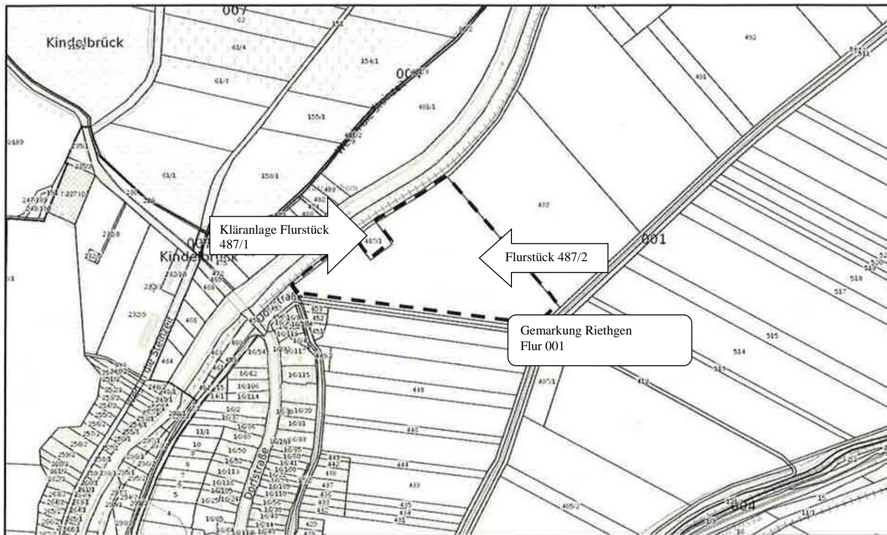
Übersichtslageplan zum Geltungsbereich des vorhabenbezogenen Bebauungsplanes der Gemeinde Riethgen für das Sonstige Sondergebiet (SO) zur Errichtung einer Photovoltaik-Freiflächenanlage
